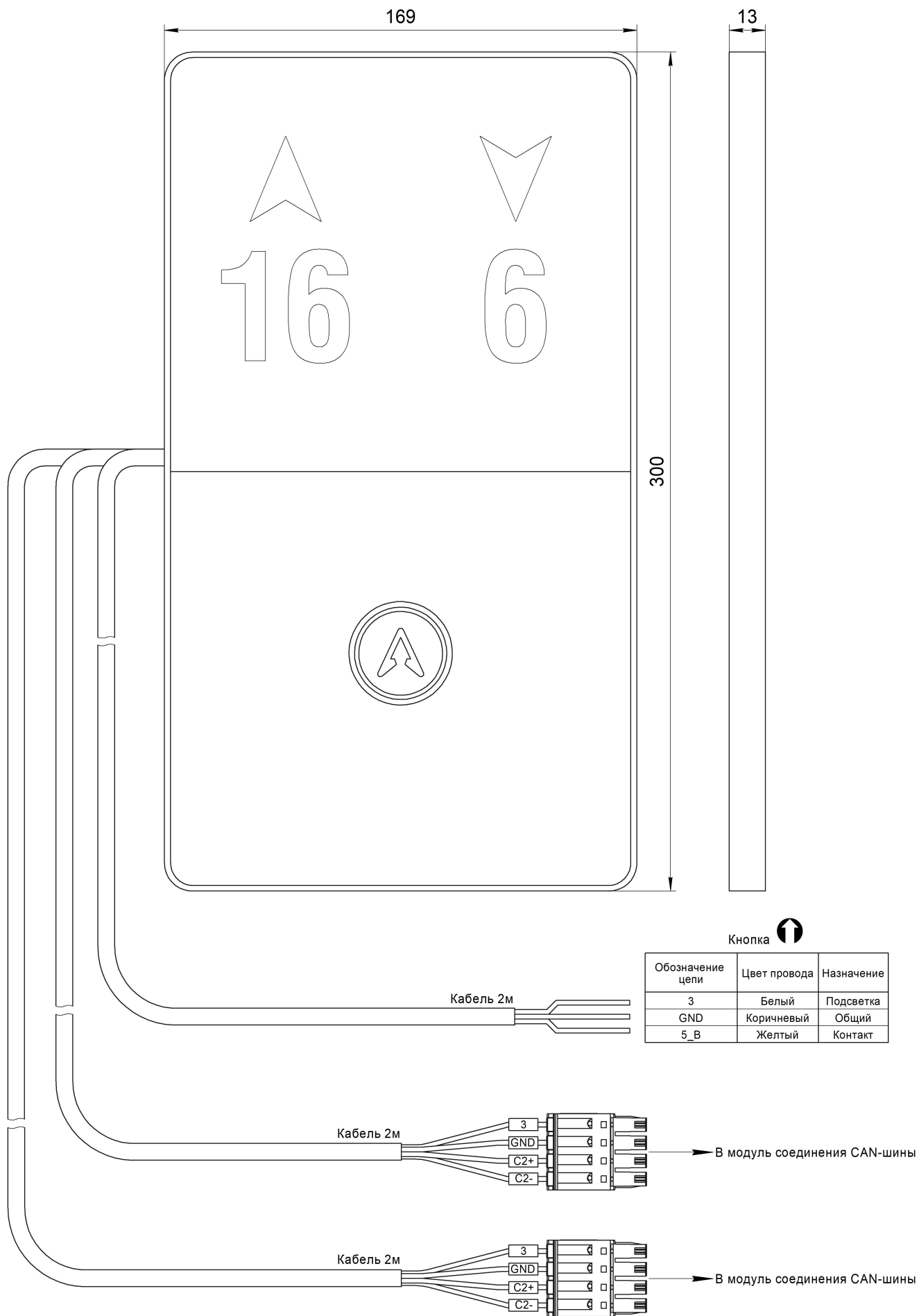
Рис.1 Внешний вид Вызывной пост ОНИКС НШЕК.468381.023
